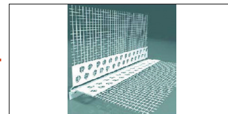
Barra rompigoccia in PVC a due scalini
