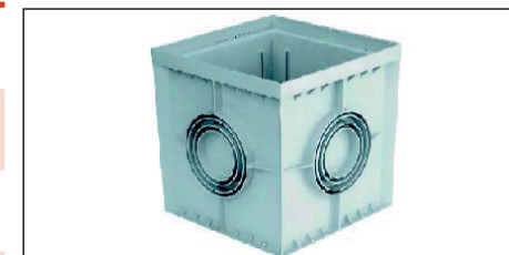
Pozzetto in PVC
