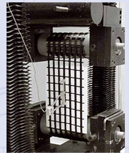
Prova di laboratorio per calcolare la resistenza della geogriglia alla massima trazione (valore T_{ult} )
