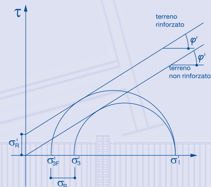
coesione apparente nel caso di terreno rinforzato
