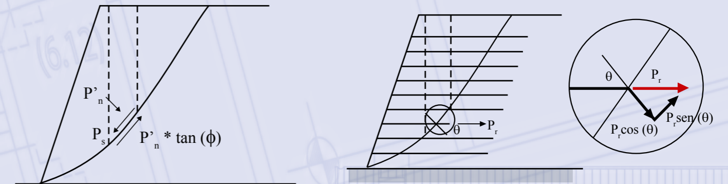
Attivazione della resistenza a trazione del rinforzo quando intercettato dalla curva di scivolamento
