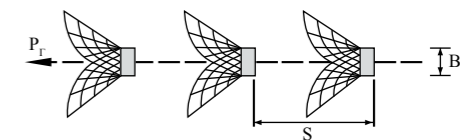
Schema di comportamento di una geogriglia per la definizione di f_{ds} e f_b
