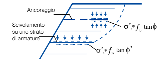
Forme di interazione tra il rinforzo sintetico e il terreno
